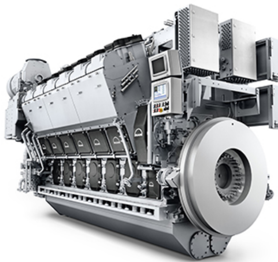
最新游轮订单中包含的MAN 51/60DF（上）和32/44CR发动机
